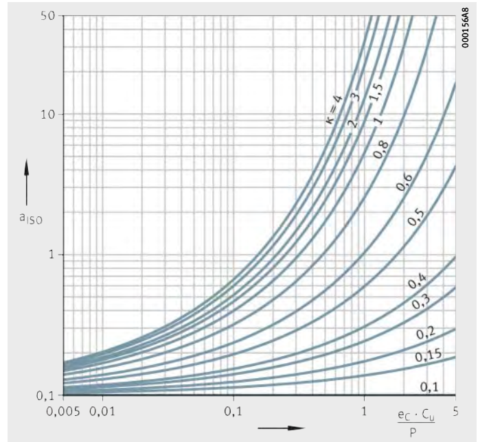
Figura 4 Coeficiente de duración de vida a_{ISO} para rodamientos radiales de rodillos
