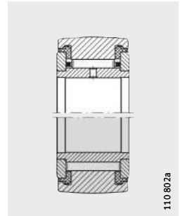
NATR..-PP (perfil INA) NATV..-PP optimizado)
