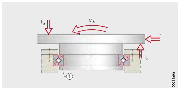
Figura 2 Rodadura con un rodamiento de rodillos cruzados
