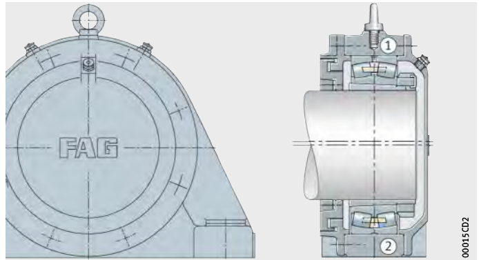
Figura 31 Soporte de apoyo BND para rodamientos con agujero cónico y manguito de fijación (obturbación de laberinto), ejecución A
