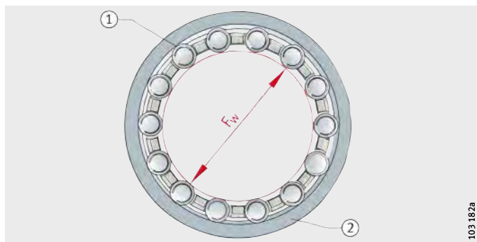
Figura 2 Círculo inscrito
