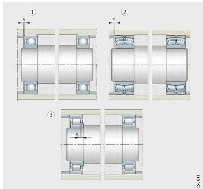
Figura 13 Rodaduras flotantes
