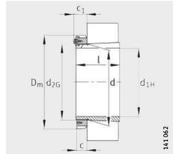
Conicidad 1:12 (conicidad 1:30 para H240), grapa de seguridad MS30
