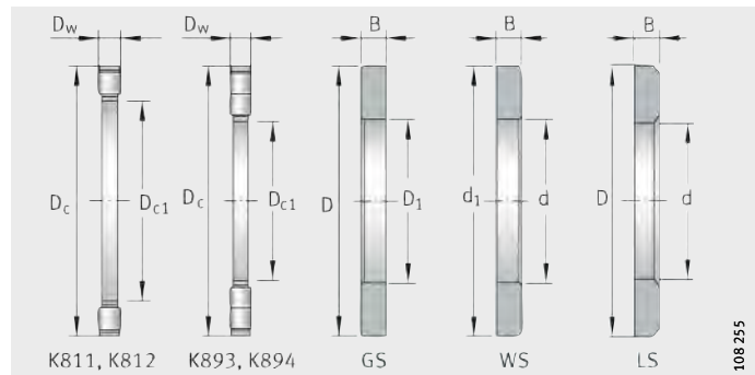
Figura 1 Componentes del rodamiento
