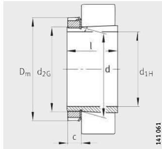
Conicidad 1:12 (conicidad 1:30 para H240 y H241) chapas de seguridad MBL y MBL
