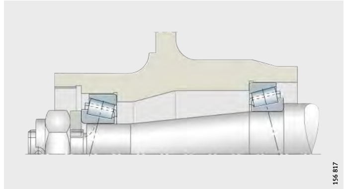
Figura 29 Rodadura ajustada
