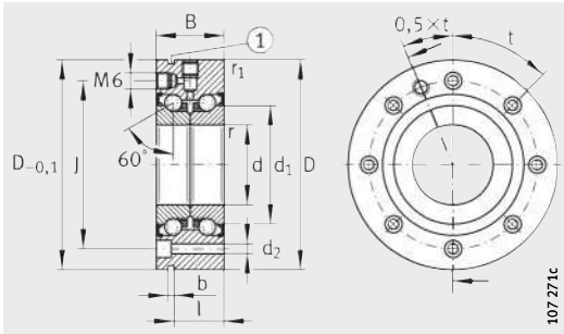
ZKLF.-2Z, ( 60 \text{ mm} \leq d \leq 100 \text{ mm} ) ① Ranura de desmontaje
