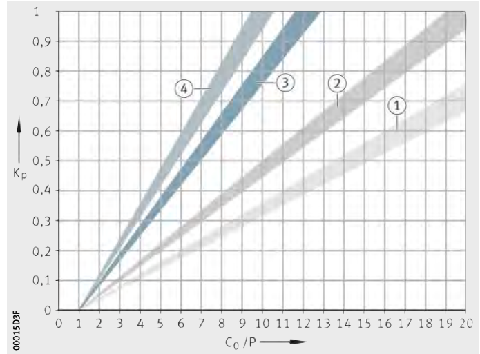
Figura 10 Factor K_p para rodamientos
