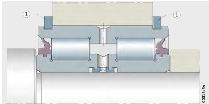
Figura 22 Rodamientos fijos
