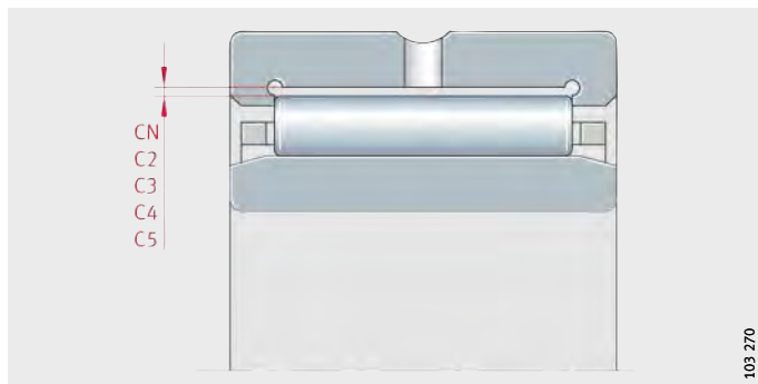
Figura 1 Juego radial
