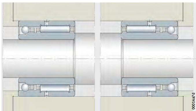
Figura 3 Dos rodamientos dispuestos uno contra otro
