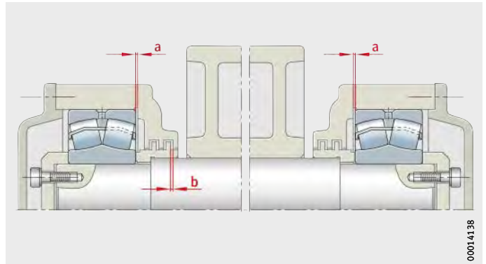
Figura 30 Rodadura flotante
