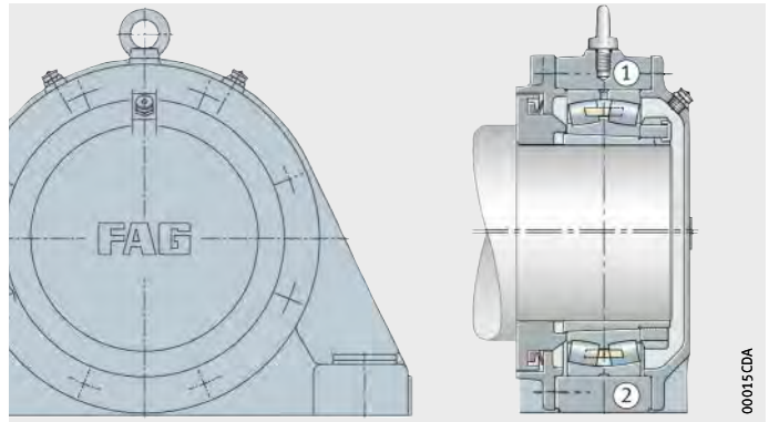
Figura 37 Soporte de apoyo BND para rodamientos con agujero cónico y manguito de fijación y para eje con resalte de apoyo (obturación Taconite), ejecución A
