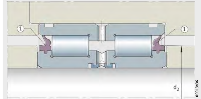
Figura 2 Apoyo de los anillos obturadores
