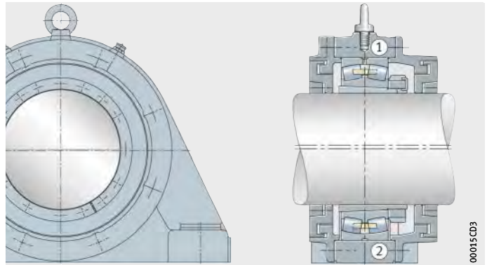
Figura 32 Soporte de apoyo BND para rodamientos con agujero cónico y manguito de fijación (obturbación de laberinto), ejecución B
