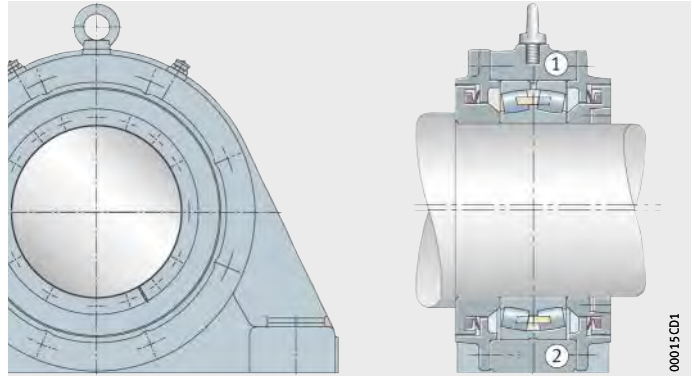
Figura 30 Soporte de apoyo BND para rodamientos con agujero cilíndrico (obturbación Taconite), ejecución B
