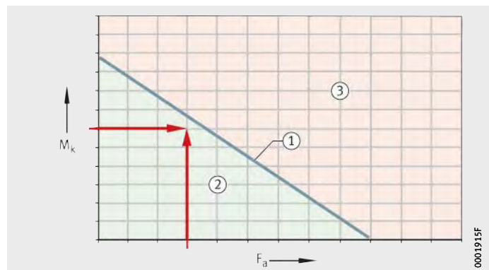
Figura 2 Diagrama de carga estática límite (Ejemplo)
