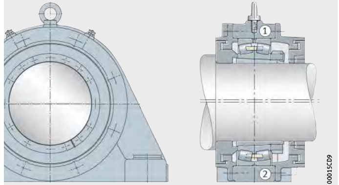
Figura 36 Soporte de apoyo BND para rodamientos con agujero cónico y manguito de fijación y para eje con resalte de apoyo (obturación de laberinto), ejecución B
