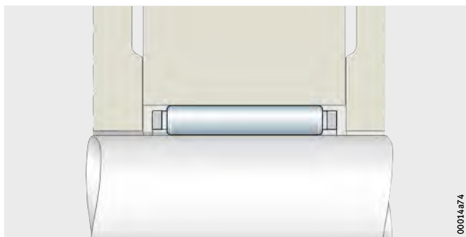
Figura 2 Seguridad axial mediante la construcción anexa
