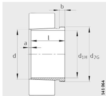
AH240 y AH241 conicidad 1:30
