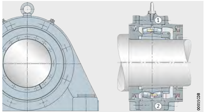
Figura 38 Soporte de apoyo BND para rodamientos con agujero cónico y manguito de fijación y para eje con resalte de apoyo (obturación Taconite), ejecución B
