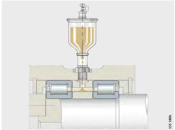
Figura 17 Lubricación por goteo de aceite (representación esquemática)
