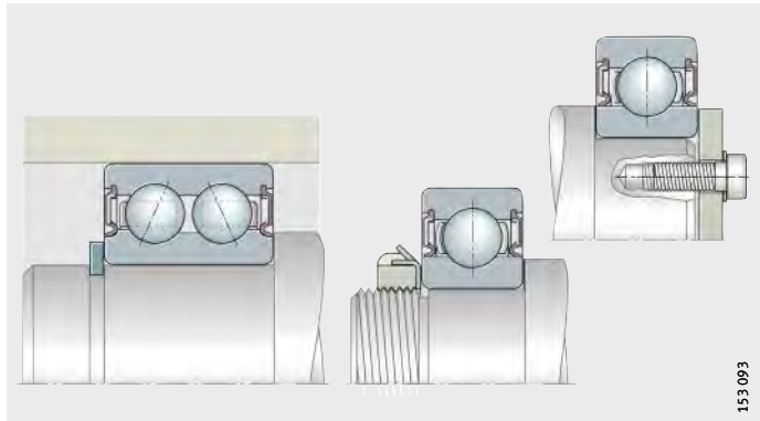
Figura 21 Rodamientos libres
